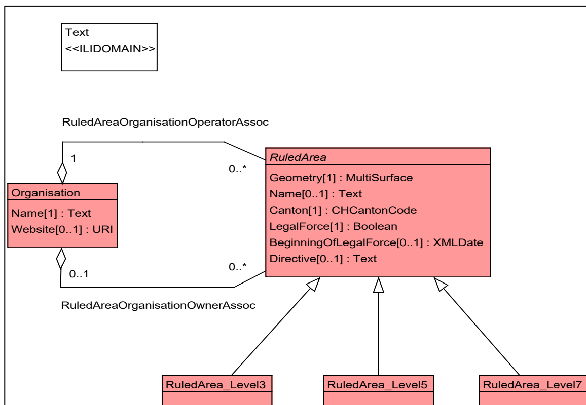
Abbildung 4: UML-Klassendiagramm Thema «SupplySecurity_RuledAreas»; die Datenerhebung der Netzebene 3 und 5 ist optional.
